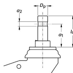
Kastor dengan Solid Stem Fitting System (akhirian SFI6)
