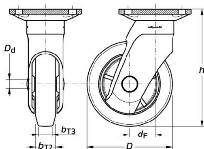
SIJ-100-P & SIJ-127-P Swivel Castors
